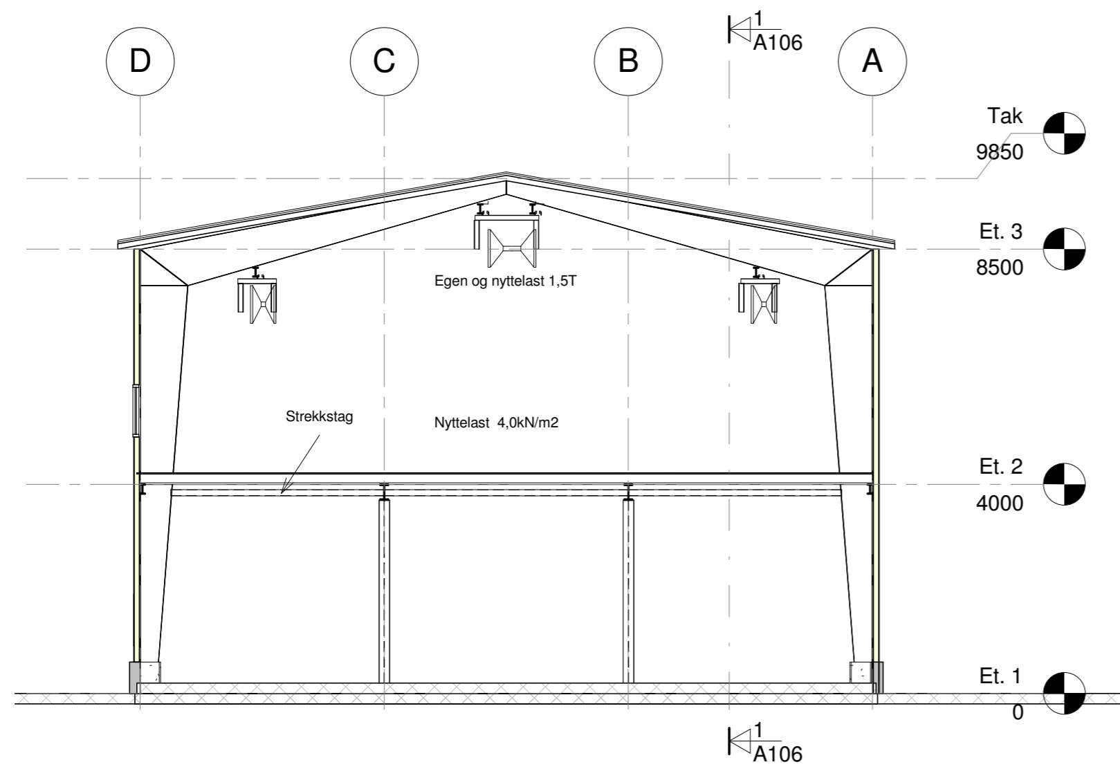
Snitt 2 1 : 100
