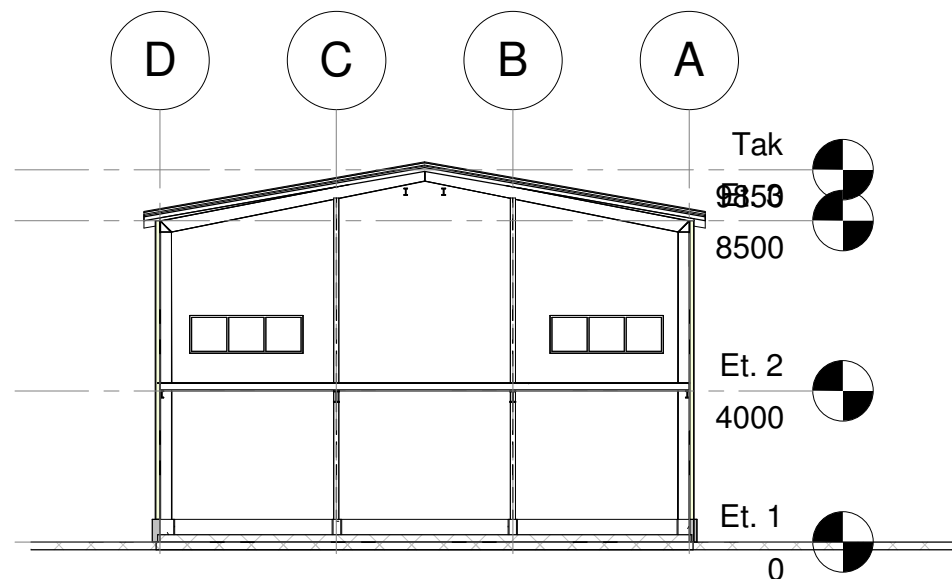
Snitt akse 7 1 : 200
