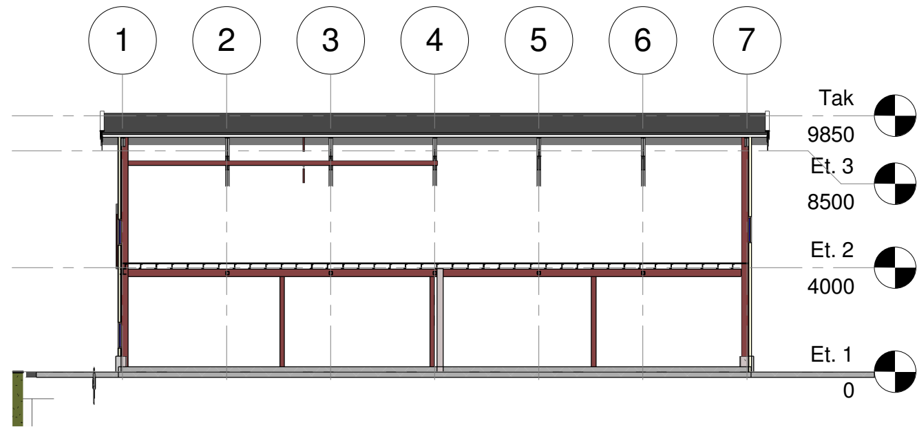
Section 3 1 : 200
