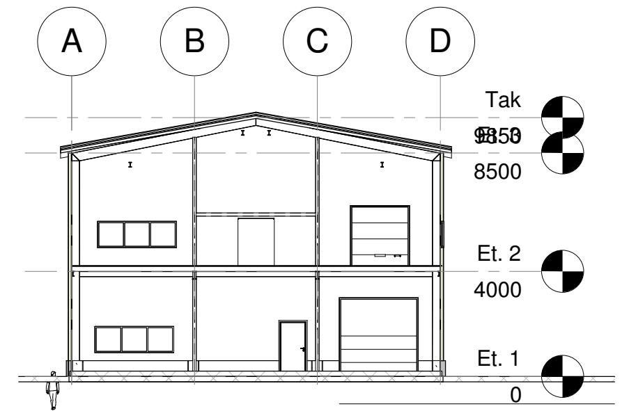
Snitt akse 1 1 : 200
